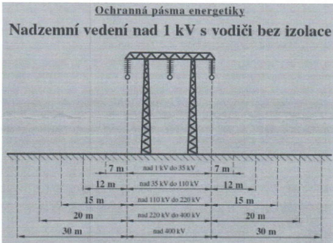
Obrázek 1: Přehled velikosti ochranných pásem
