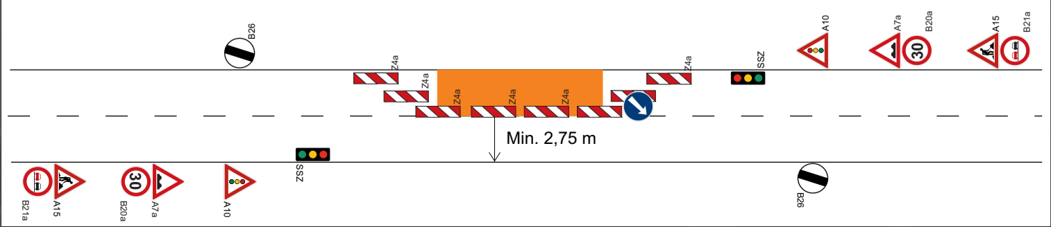
Detail pracovního místa - dle upraveného schéma B/6 bude realizováno dle vyznačených úseků.
